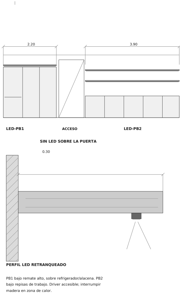
D-M01 / MADERA Y LED EN COCINA
