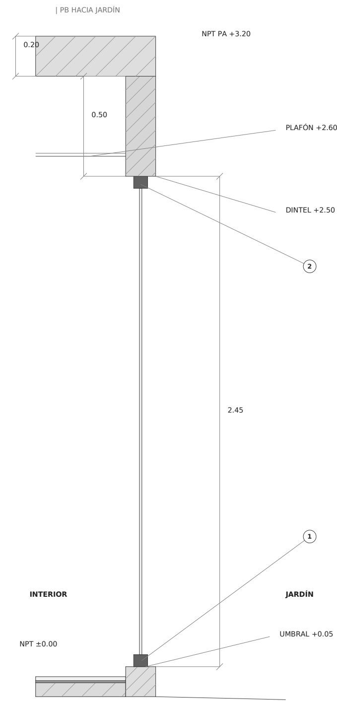
D-V01 / SECCIÓN GENERAL
